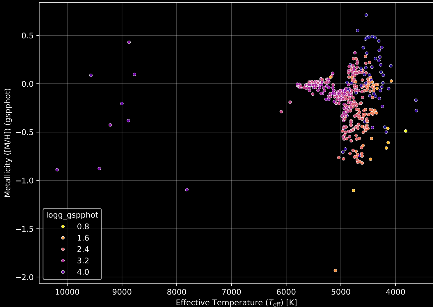
APOGEE DR17 Field: [240+08] Stellar Population Parameters (n= 467)
